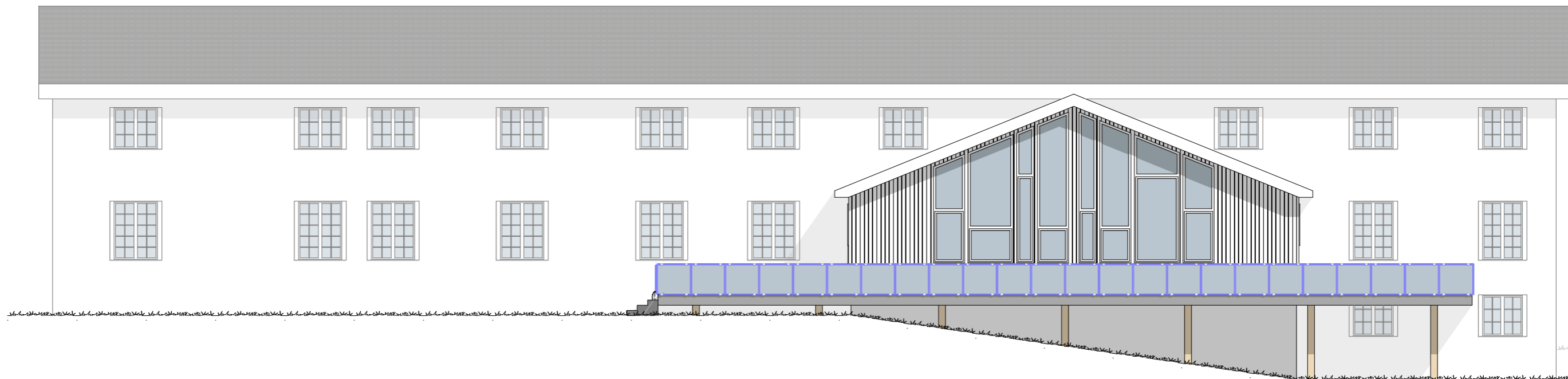
1:125 Fasade Nord
